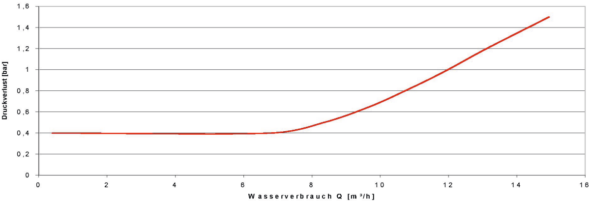
MVR AC 1" Magnetventil VMF5 50305 (ohne Druckregler)
