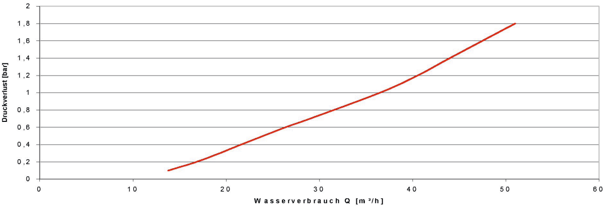
MVR AC 2" Magnetventil VM I5 50307 (ohne Druckregler)
