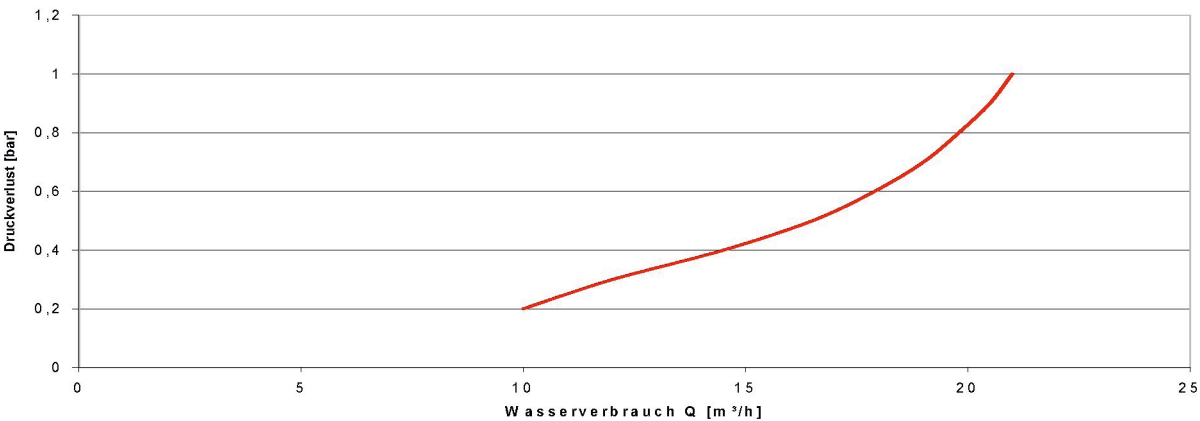
MVR AC 1 1/2" Magnetventil VMH5 50306 (ohne Druckregler)
